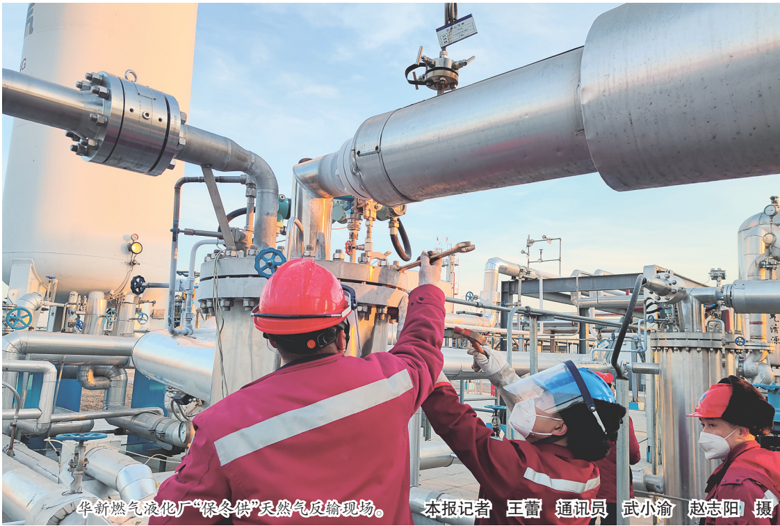
华新燃气液化厂“保冬供”天然气反输现场。
